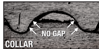
HuckBolt®
